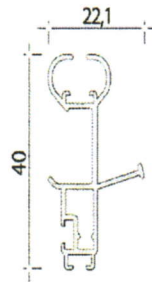
Griffschiene
